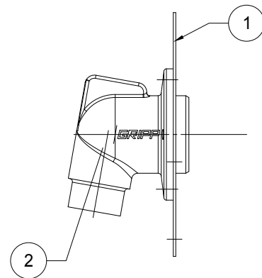
Raccord à souder
